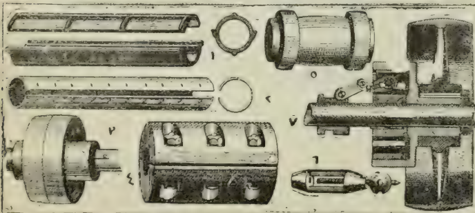
(میل بیانغری)
